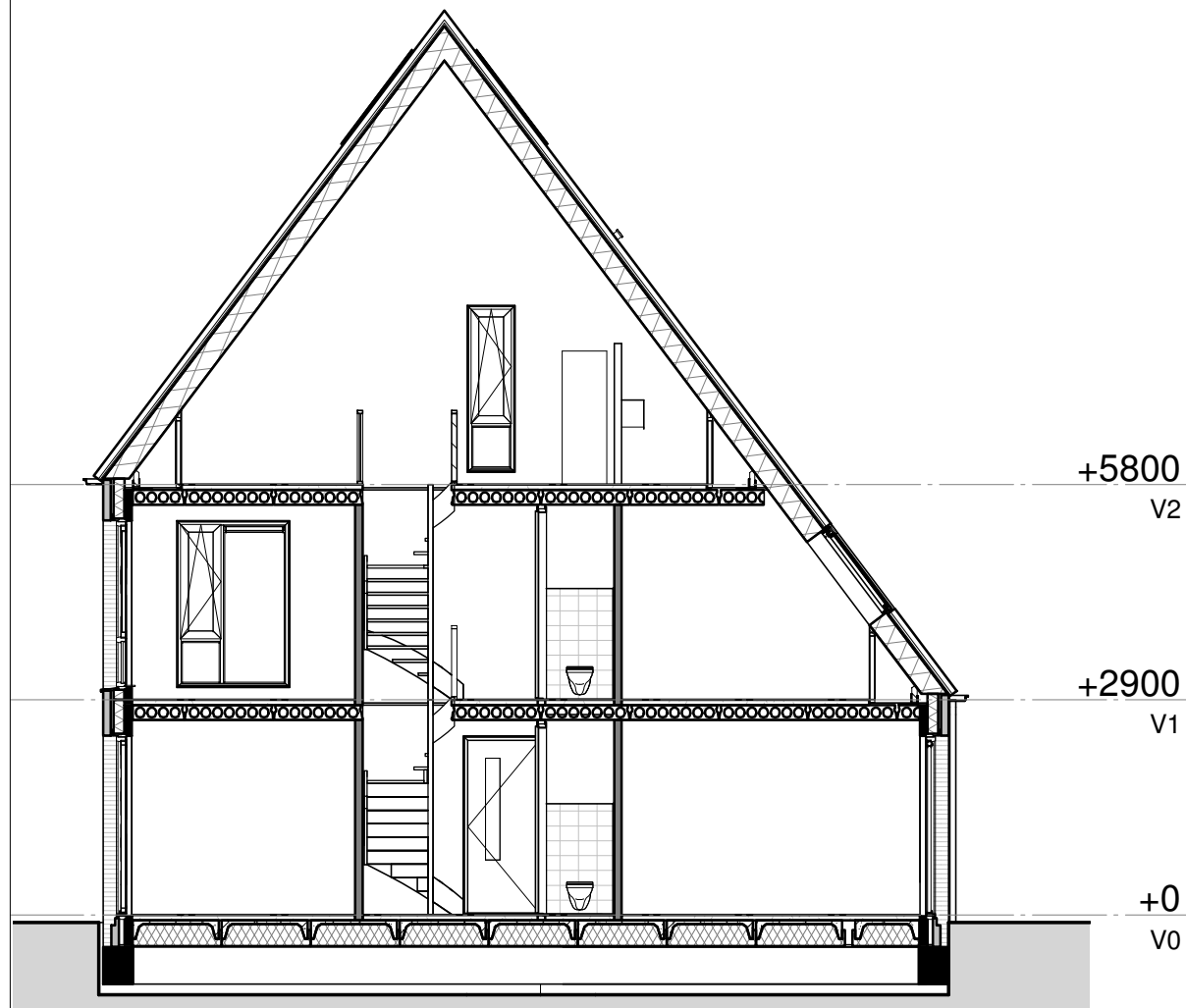
Doorsnede bouwnr: 1-2, 5-6, 30-31, 40
